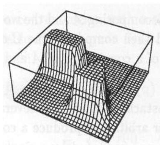
La funzione potenziale repulsivo
