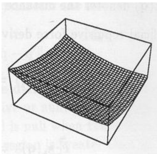
La funzione potenziale attrattivo iperbolica
