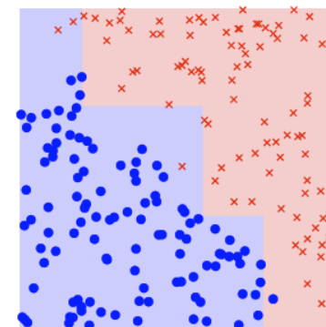
\mathcal{S}_{10}
