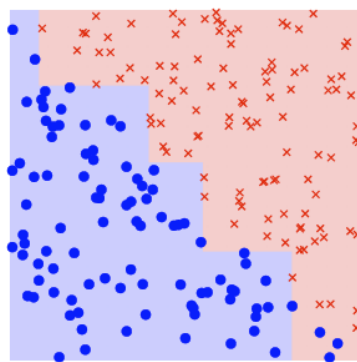
\mathcal{S}_3
