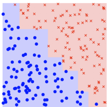
\mathcal{S}_6
