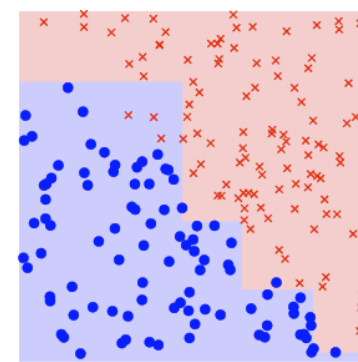
\mathcal{S}_5
