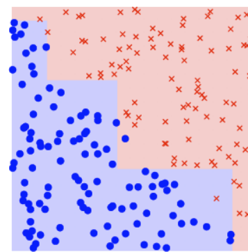
\mathcal{S}_4
