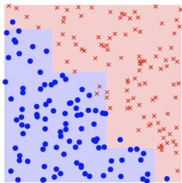
\mathcal{S}_1
