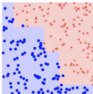
\mathcal{S}_7
