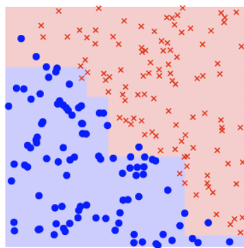
\mathcal{S}_2
