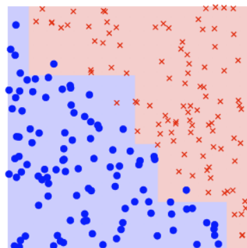
\mathcal{S}_8
