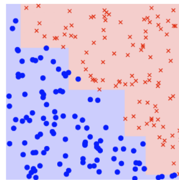
\mathcal{S}_9
